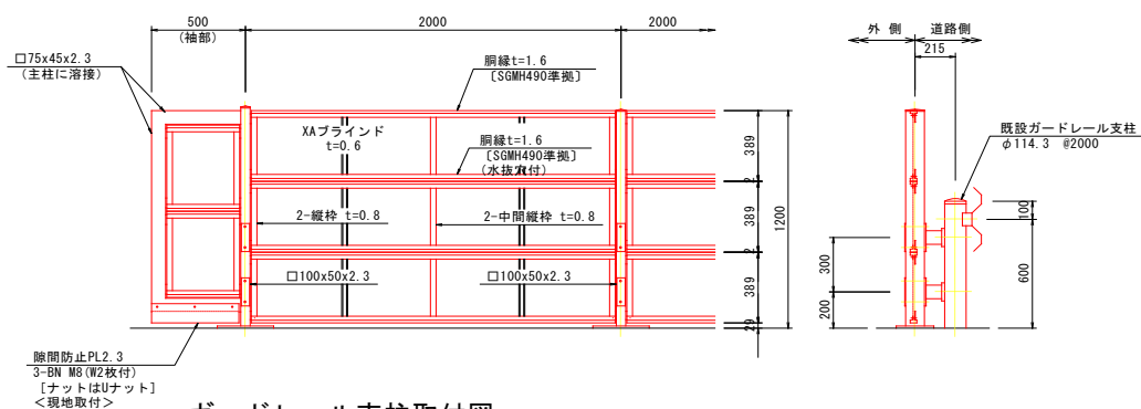
ガードレール支柱取付図
